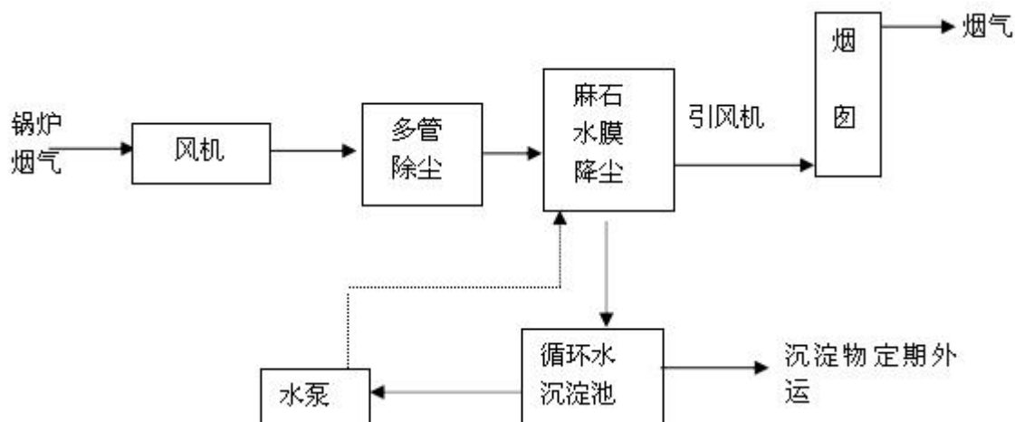
图 3-5 锅炉烟气处理流程示意图
