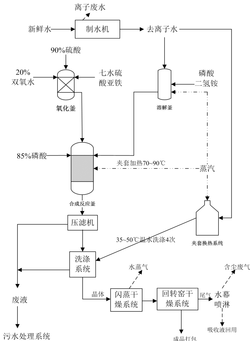
图 3-3 磷酸铁生产工艺及产污环节图
