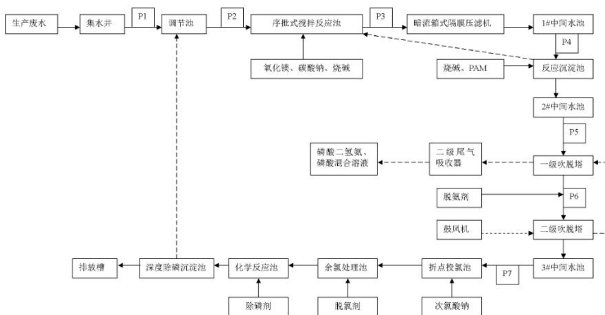
图 3-4 污水处理工艺流程图
