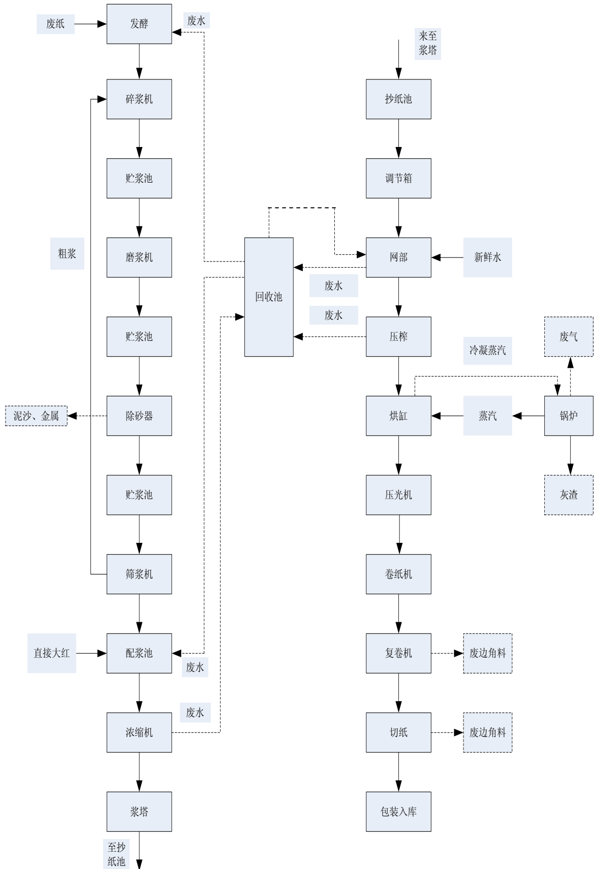
图 3-2 鞭炮纸工艺流程及产污节点
