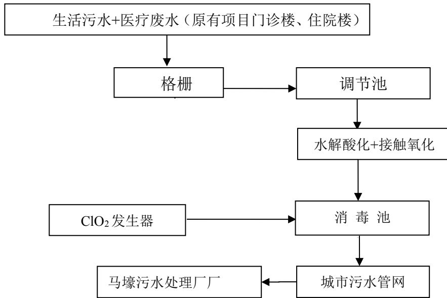
图 3-4 医院污水处理流程图
