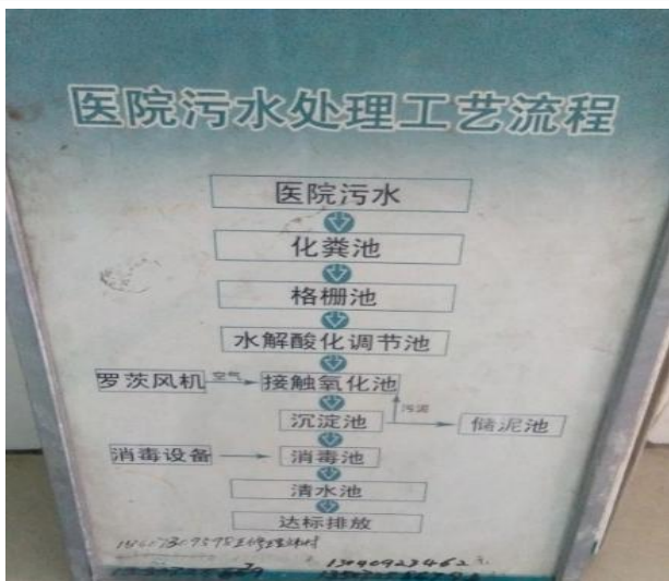
污水处理工艺流程图
