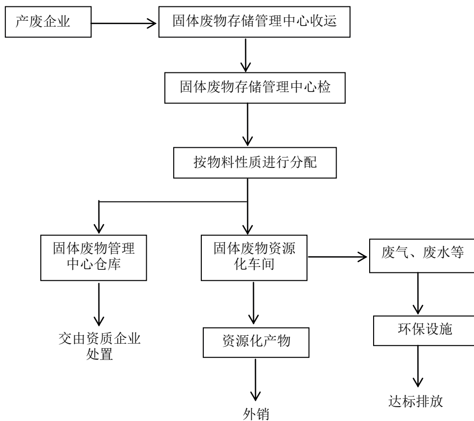
图 2.11-1 工程技术路线
