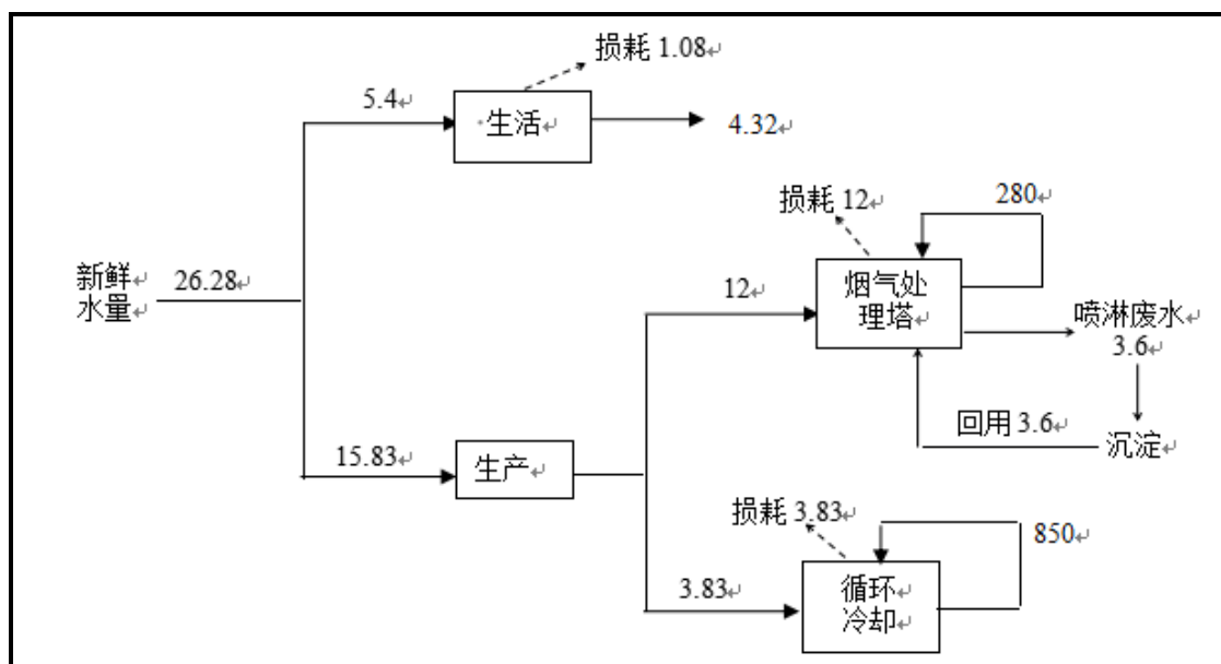
图 2.12-1 项目水平衡图 单位: m 3 /d
