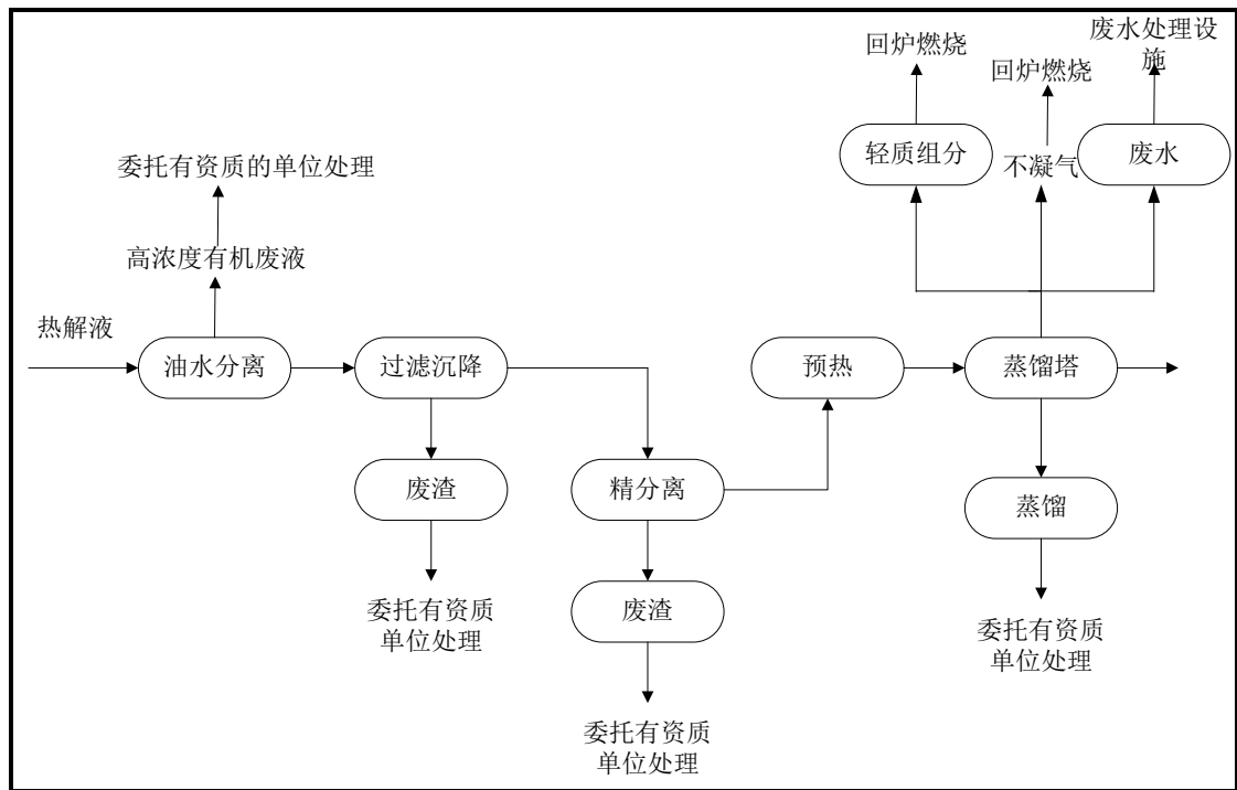
图 3.7-1 热解液精炼工艺流程及产污环节
