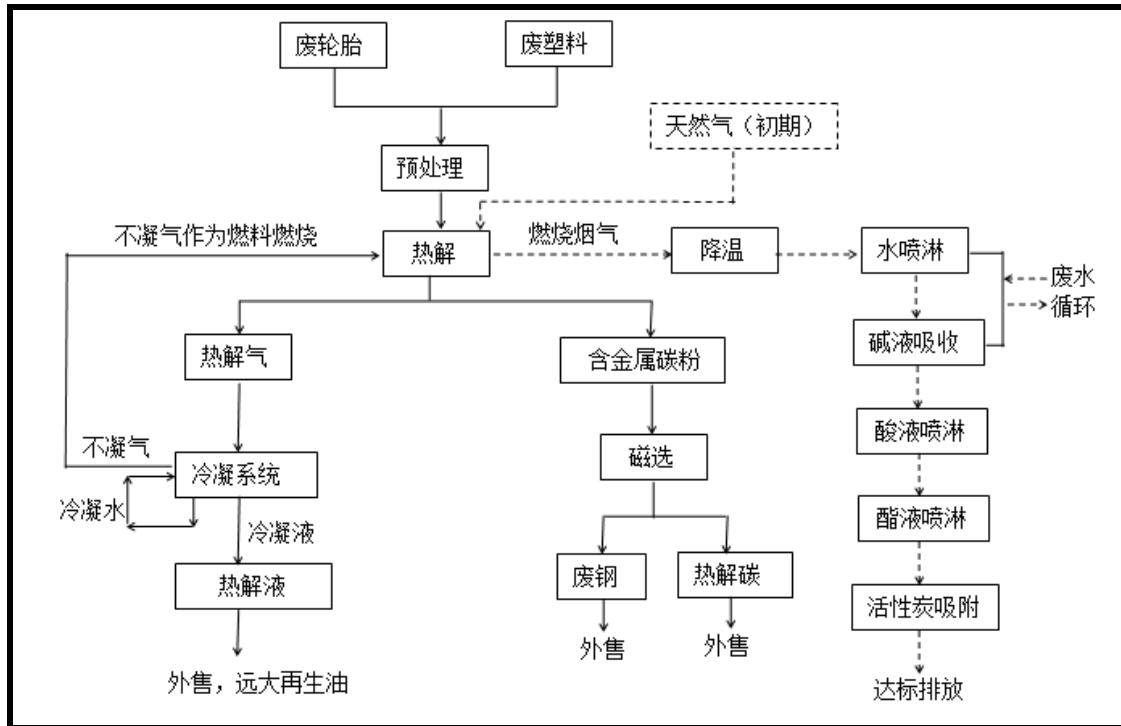
图 2.11-4 废轮胎、废塑料资源化利用工艺及产污节点图
