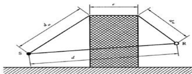
图 6.3-3 双绕射情景示意图
