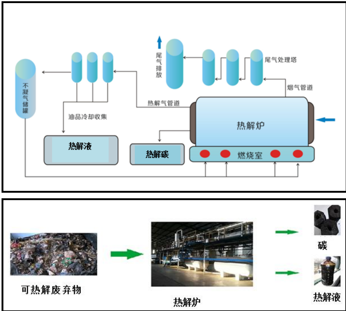
图 2.11-2 低温热解工艺流程图
