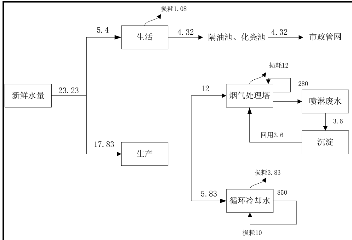
图 5.1-1 变更后全长水平衡图 单位: \text{m}^3/\text{d}
