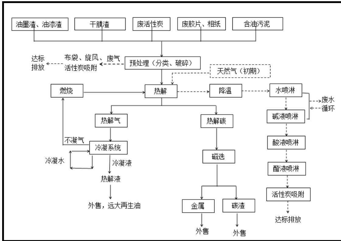
图 2.11-3 固体废物资源化利用工艺流程及产污节点图
