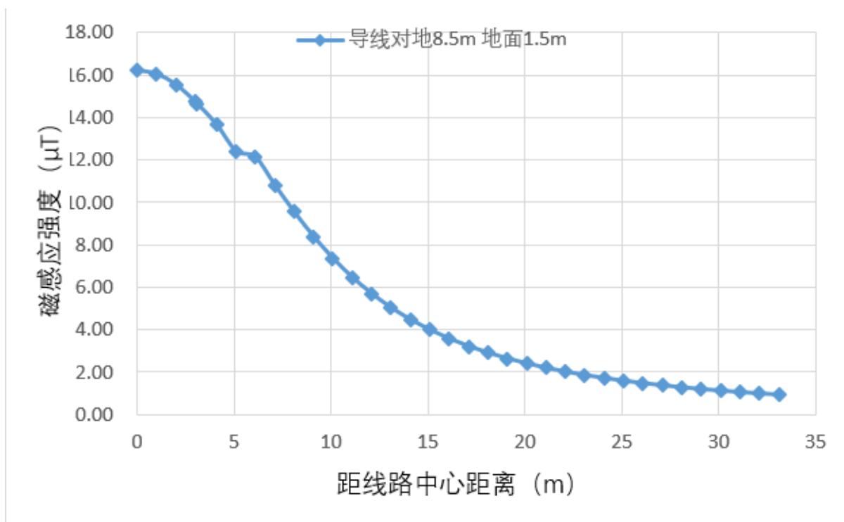
图 19 110kV 单回线路工频磁场预测结果
