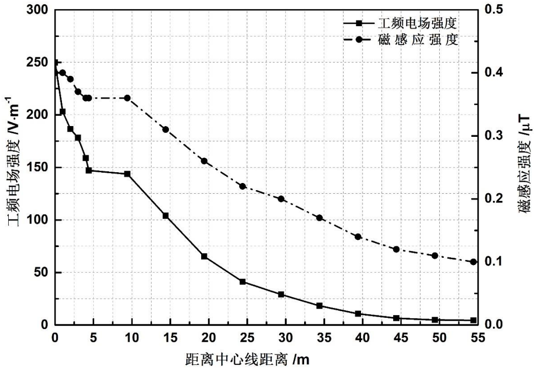
图 15 110kV 图周线、110kV 图湘线工频电场、工频磁场随距离衰减趋势
