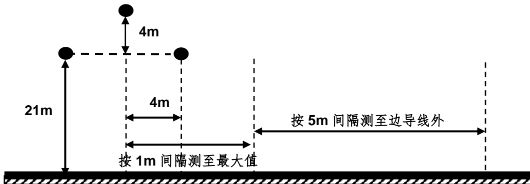
图 12 110kV 滨下六线电磁衰减断面监测示意图
