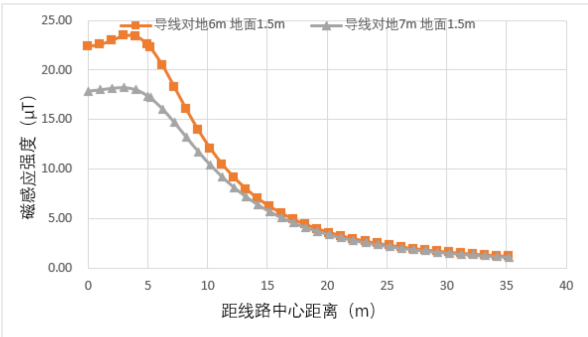
图 20 110kV 双回线路工频磁场预测结果
