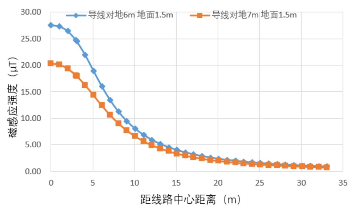
图 18 110kV 单回线路工频磁场预测结果
