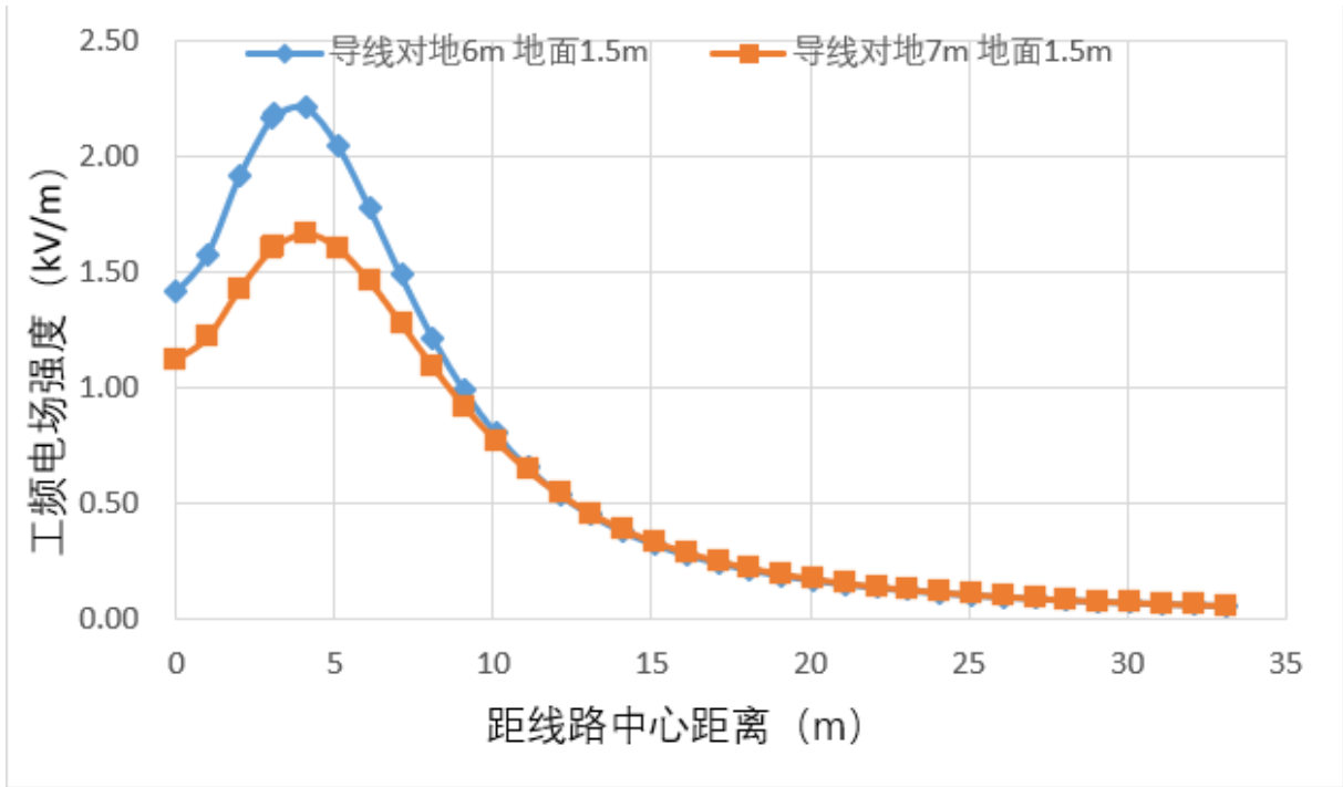
图 17 110kV 单回线路工频电场预测结果
