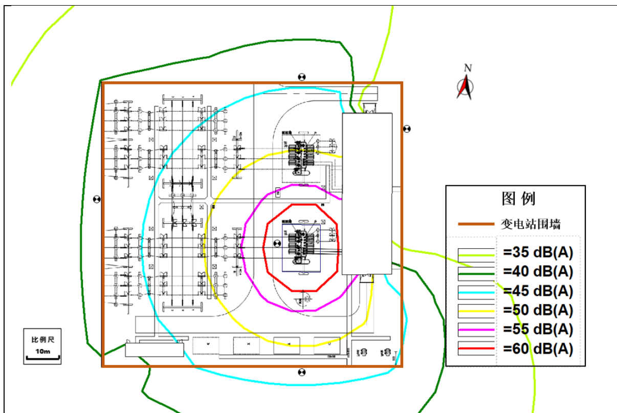
图 9 屈原河市 110kV 变电站本期规模噪声预测等值线图
