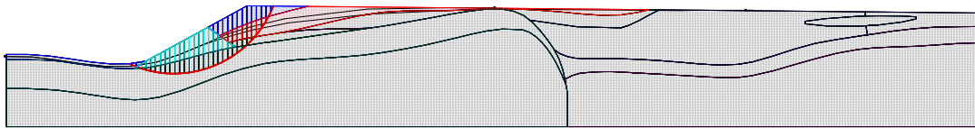
图 7-5 1-1' 剖面堆积坝 90m 标高最危险滑弧位置
