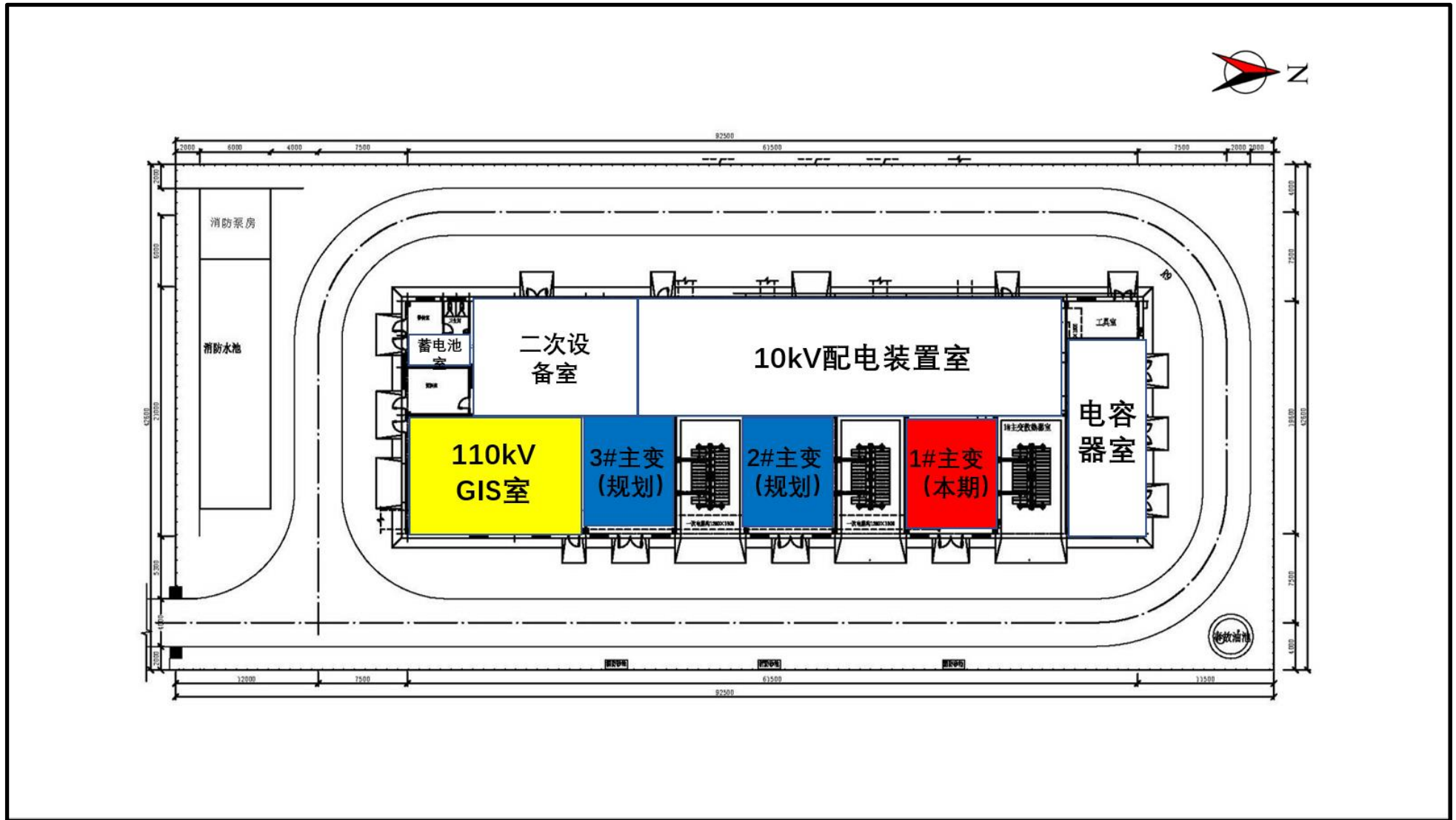
附图 2 百丈 110kV 变电站总平面布置图
