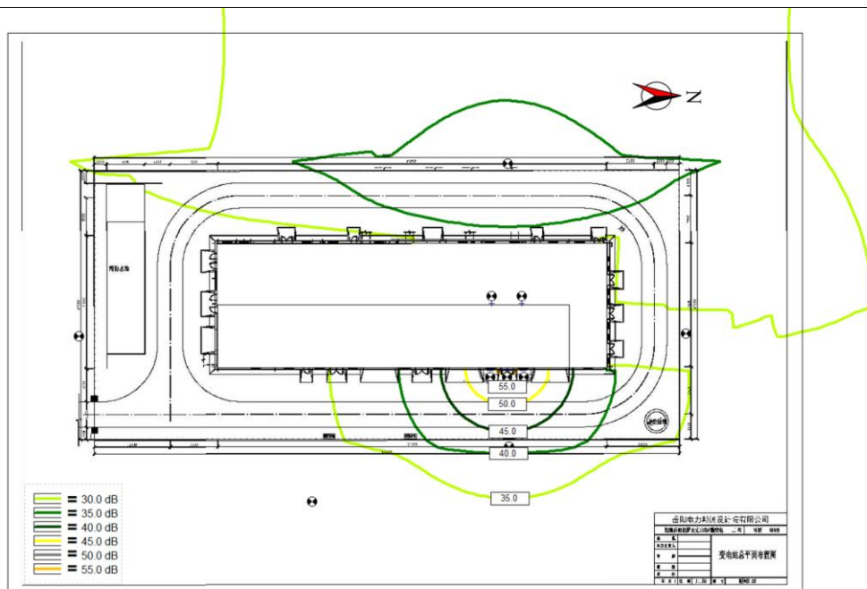
图 9 百丈 110kV 变电站本期规模噪声预测等值线图
