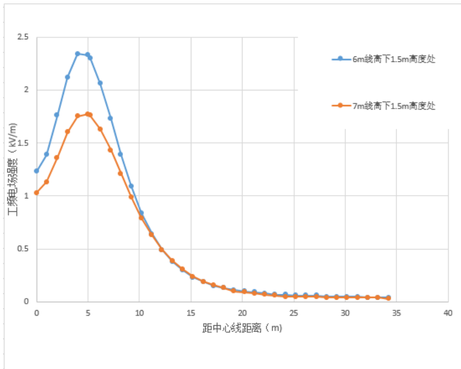
图 19 110kV 双回线路工频电场强度预测结果
