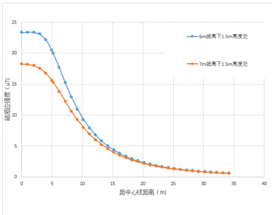
图 20 110kV 双回线路磁感应强度预测结果
