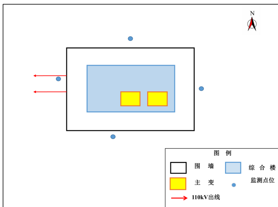
图 10 洋湖 110kV 变电站平面布置及监测点位示意图
