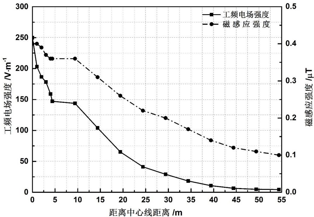
图 12 110kV 图周线、110kV 图湘线工频电场、工频磁场随距离衰减趋势
