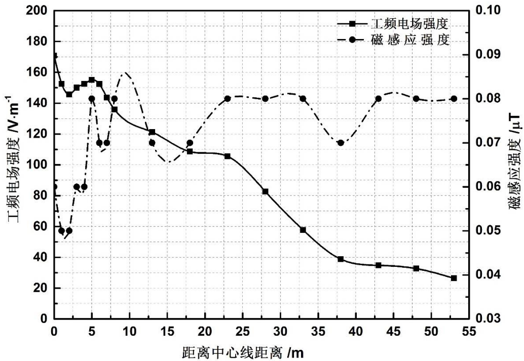
图 11 110kV 桂朴美线工频电场、工频磁场随距离衰减趋势
