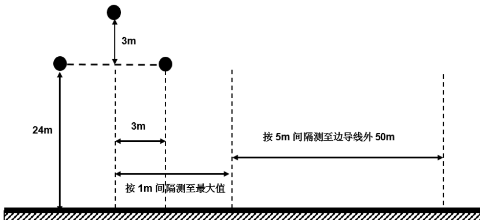
图 12 110kV 桂朴美线电磁衰减断面监测示意图
