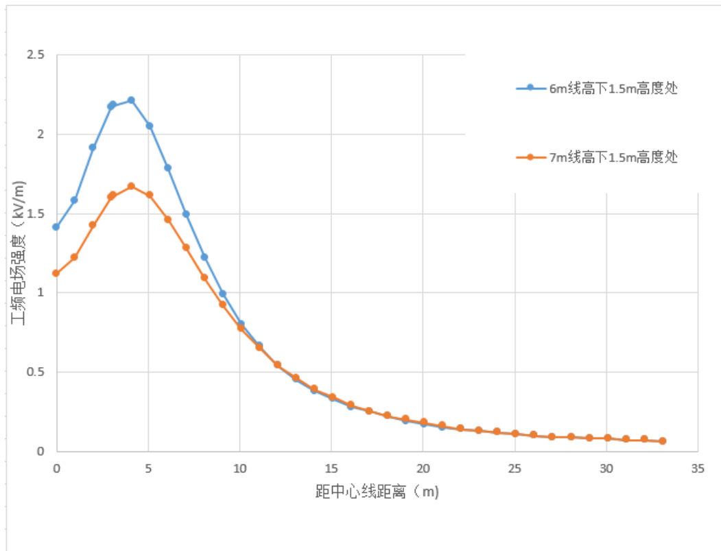
图 14 110kV 单回线路工频电场强度预测结果
