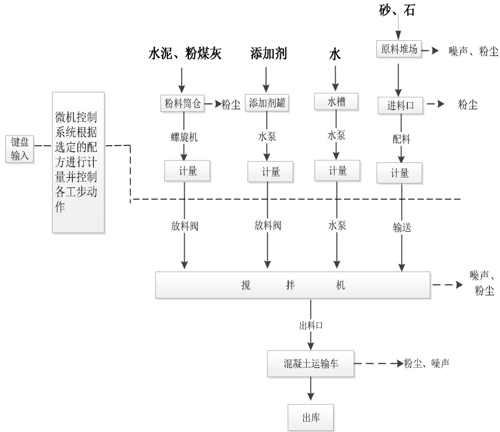
图 2-2 混凝土生产工艺流程图及产污节点图
