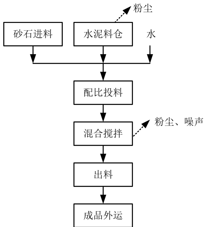
图 2-3 水稳料生产工艺流程及产污节点图
