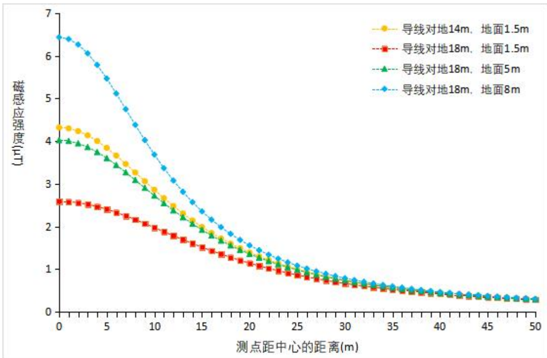
图 5 工频磁感应强度预测结果
