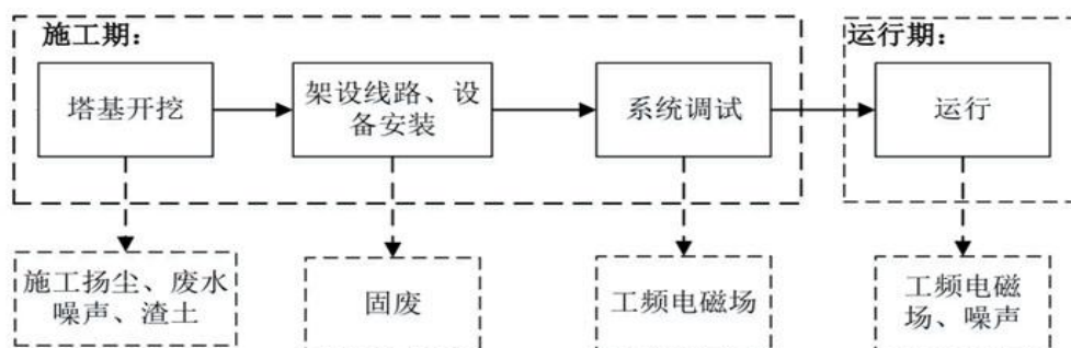
图 2-3 架空输电线路建设流程和产污节点图
