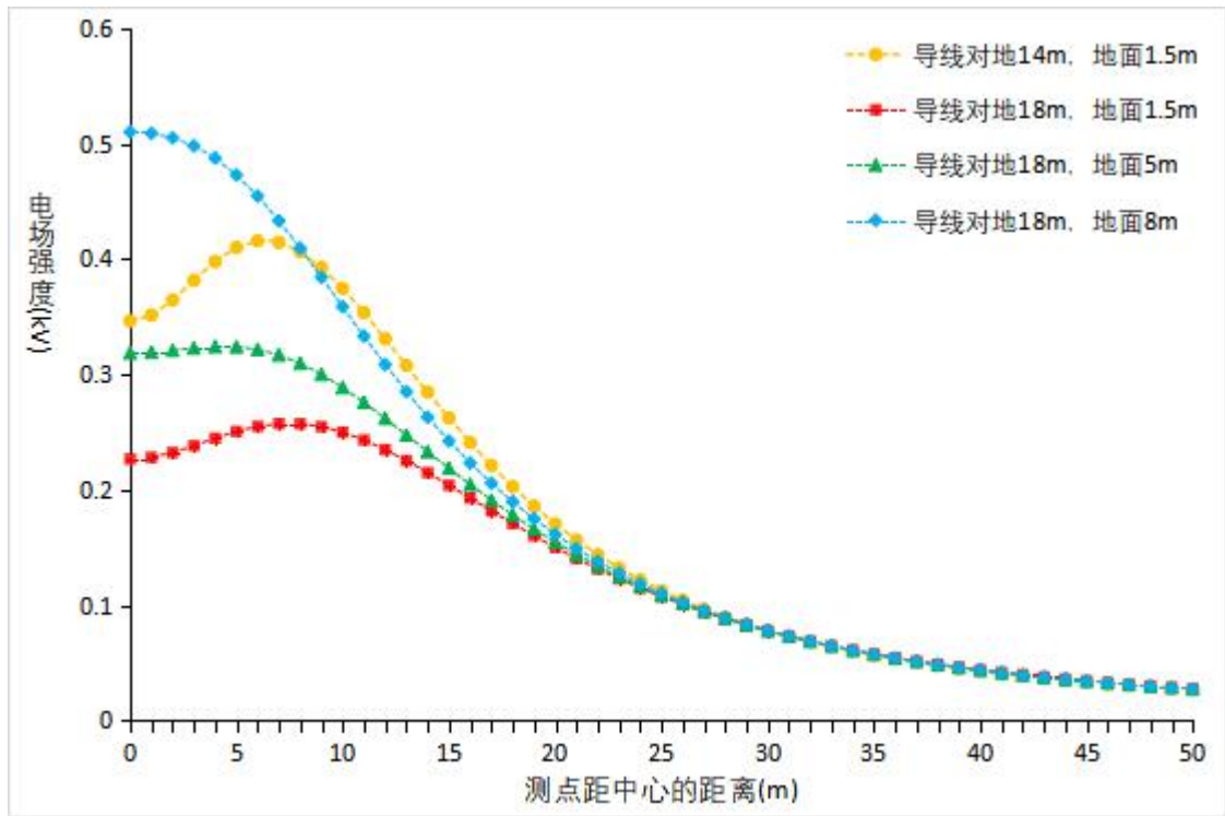
图 4 工频电场强度预测结果
