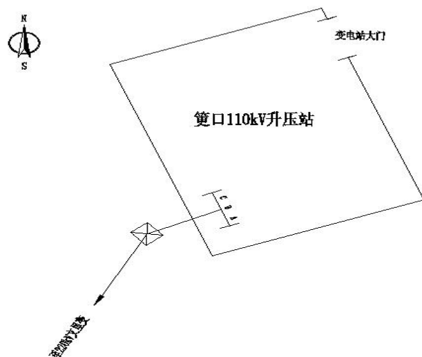
图 2-1 箕口光伏电站 110kV 升压站进出线平面布置图
