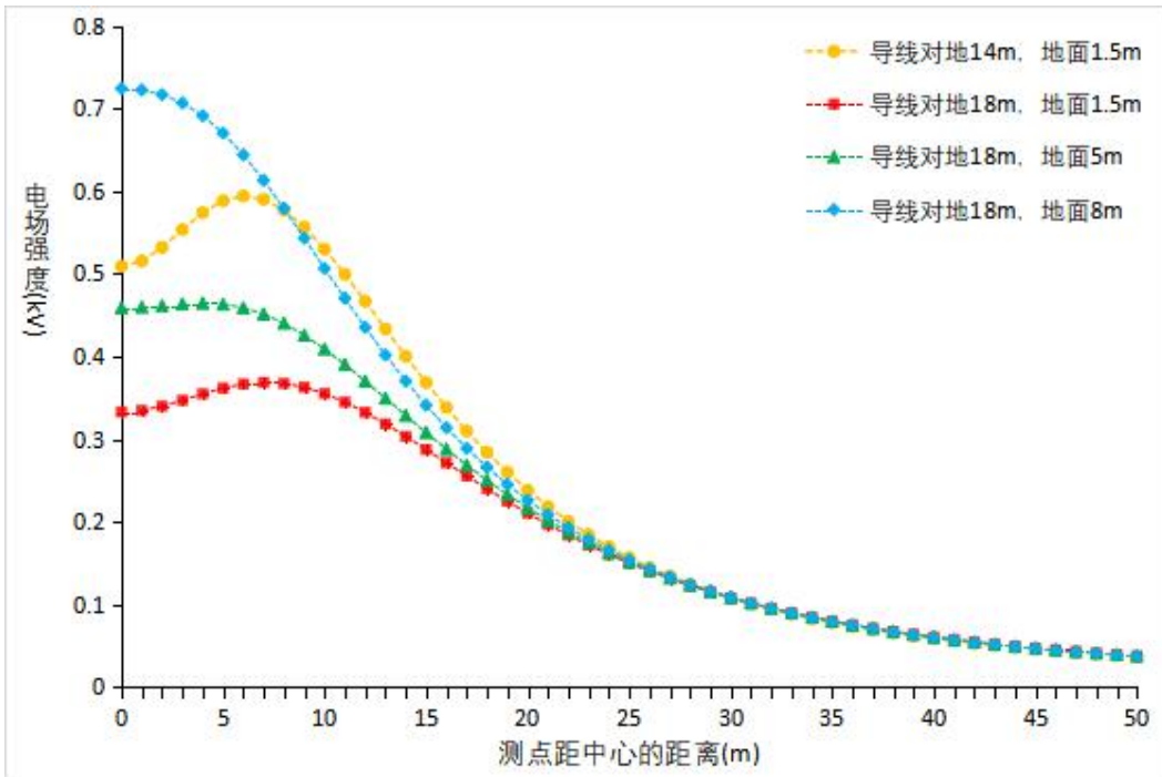
图 6 工频电场强度预测结果
