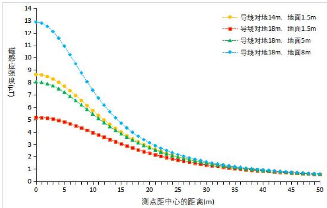
图 7 工频磁感应强度预测结果
