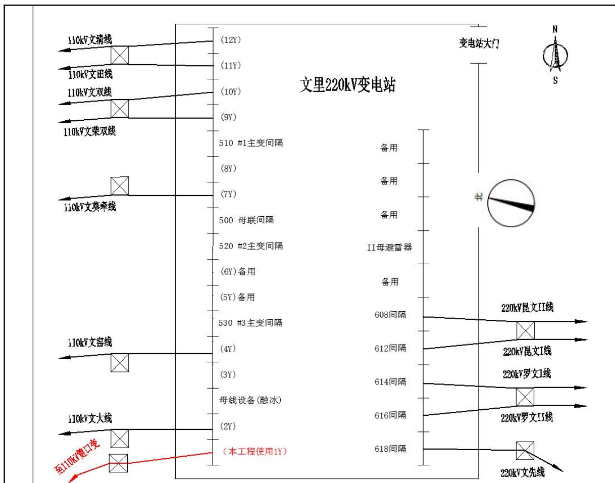
图 2-2 文里变电站进出线平面布置图
